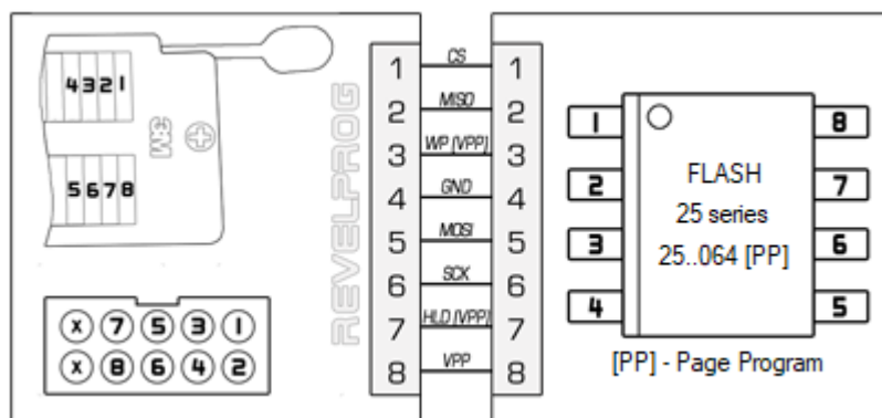
Podłączenie „1 do 1” dla pamięci FLASH SPI
